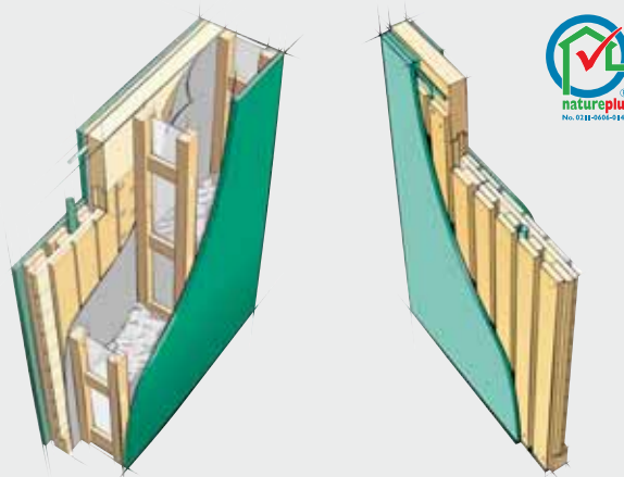
Aussenwand hoch wärmedämmt: LIGNO Fux 4S und U*psi F
