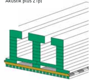
LIGNO Rippe Q3 BV (hier: Ausführung Akustik plus Z1p)
