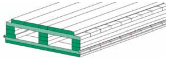
LIGNO Block Q3 Akustik BV (hier: Ausführung mit Leistenprofil)
