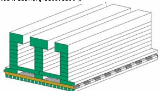
LIGNO Rippe Q3 BV (hier: Ausführung Akustik plus Z1p)
