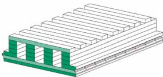
LIGNO Decke Q4
