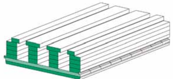
LIGNO Rippe Q4
