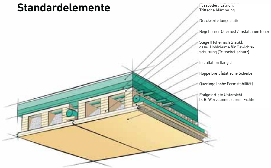
LIGNO Decke Q3
