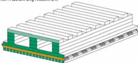
LIGNO Decke Q3 (hier: Ausführung Akustik Z1)
