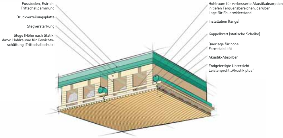
LIGNO Rippe Q3 BV (hier: Ausführung Akustik plus Z1p)
